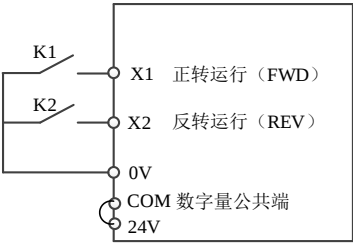
NPN型接法
