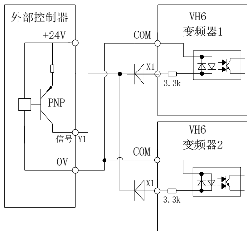
多台变频器使用外部24V电源的源型接线方法
