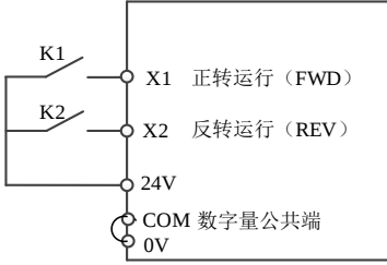
PNP型接法
