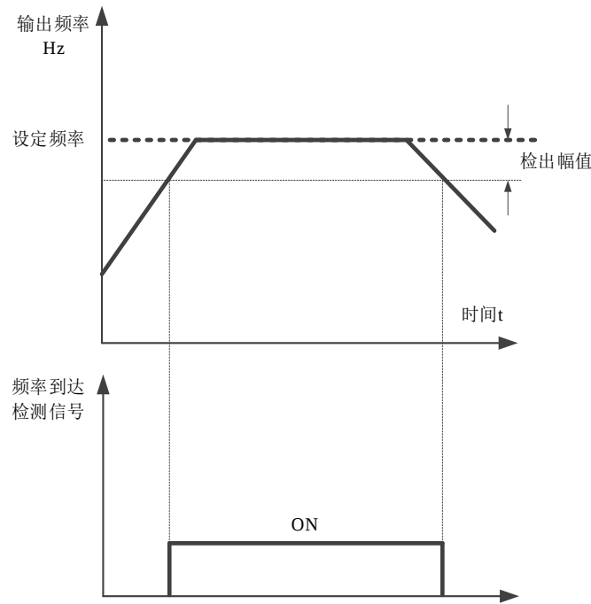
一段速曲线
